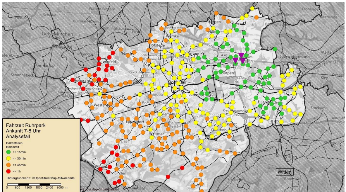
Abbildung 22: Fahrzeiten vom Ruhrpark (Werktag 7-8 Uhr, Fahrplan 2015)
