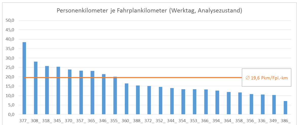
Abbildung 25: Personenkilometer je Fahrplankilometer für Linien mit >80% Fahrplanleistung in Bochum (Werktag, Analysefall 2015)
