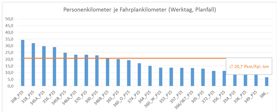
Abbildung 40: Personenkilometer je Fahrplankilometer für Linien mit >80% Fahrplanleistung in Bochum (Planfall)
