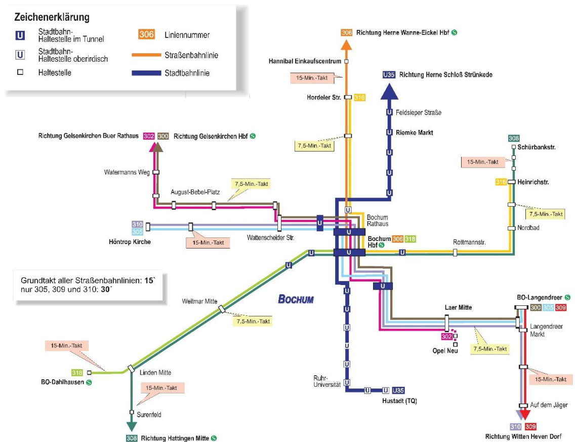
Abbildung 29: Takte und Linienwege im Straßenbahnkonzept mit 15-/30-Minuten-Takt (Quelle: BOGESTRA)
