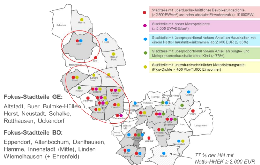
Abbildung 42: Potenzialabschätzung BOGESTRA-Bediengebiet
