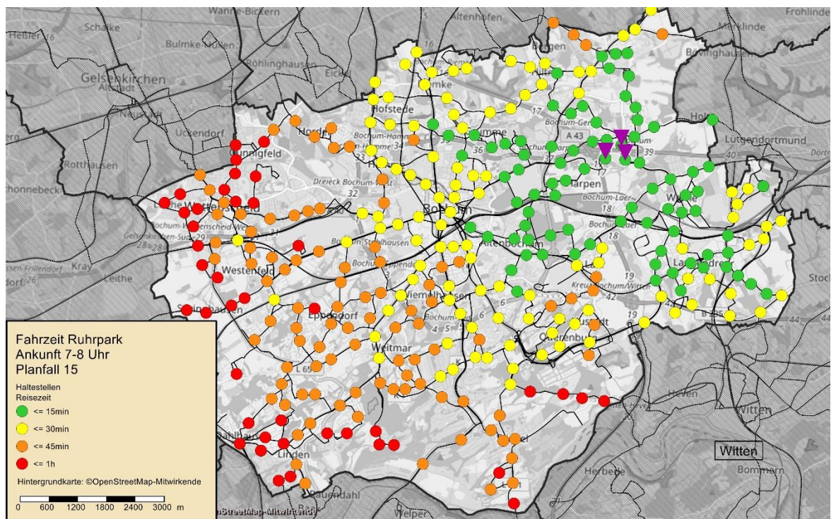
Abbildung 38: Fahrzeitdarstellung vom Ruhrpark, Werktag 7-8 Uhr, Planfall 15
