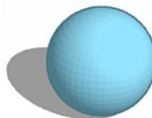
сфера
