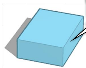
кубоид
