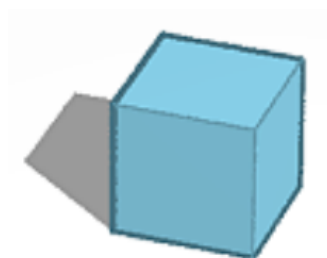
куб
