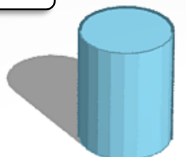
цилиндър
