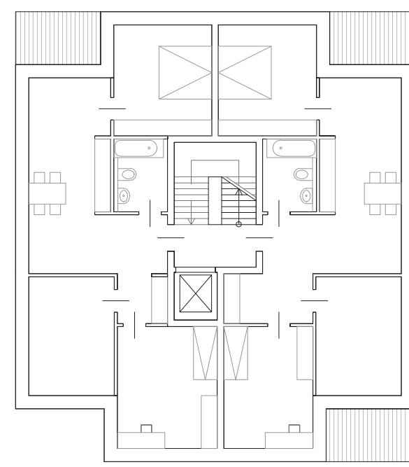
OBERGESCHOSS 1:200
