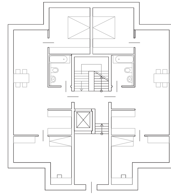
ERDGESCHOSS 1:200
