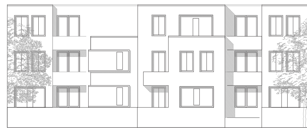
ANSICHT 1:200
